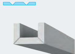
3x 90° V-Fräsungen
