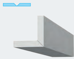
2x 90° V-Fräsungen
