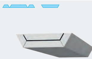
2 + 2 90° V-Fräsungen
