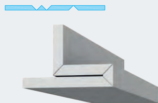
2 + 1 90° V-Fräsungen
