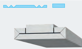
2 + 2 90° V-Fräsungen
