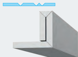
1x 45° + 1x 90° V-Fräsungen
