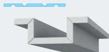
2 + 2 90° V-Fräsungen
