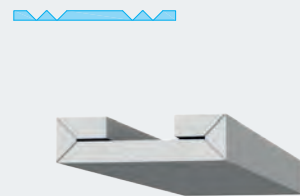
4x 90° V-Fräsungen + Plattenstreifen
